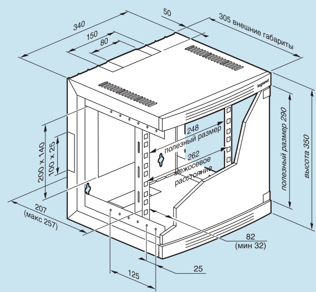
Шкаф мини XL VDI глуб. 300 мм
