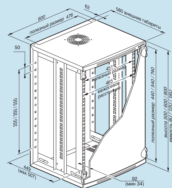
Шкафы с поворотной рамой XL VDI глуб. 600 мм
