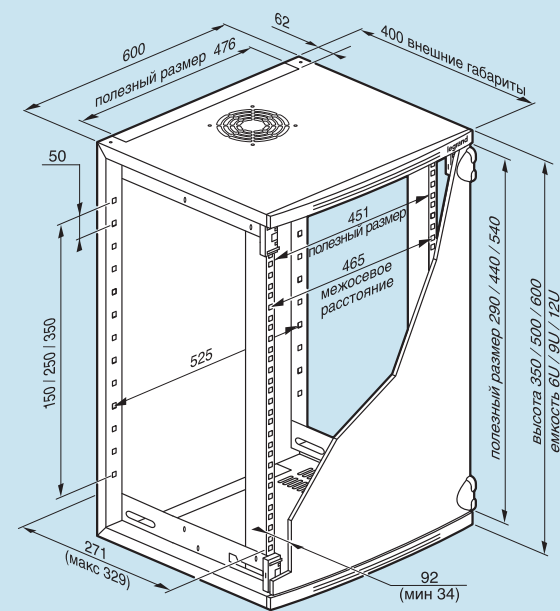
Шкафы фиксированные XL VDI глуб. 580 мм
