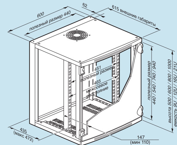
Шкафы с поворотной рамой XL VDI глуб. 600 мм
