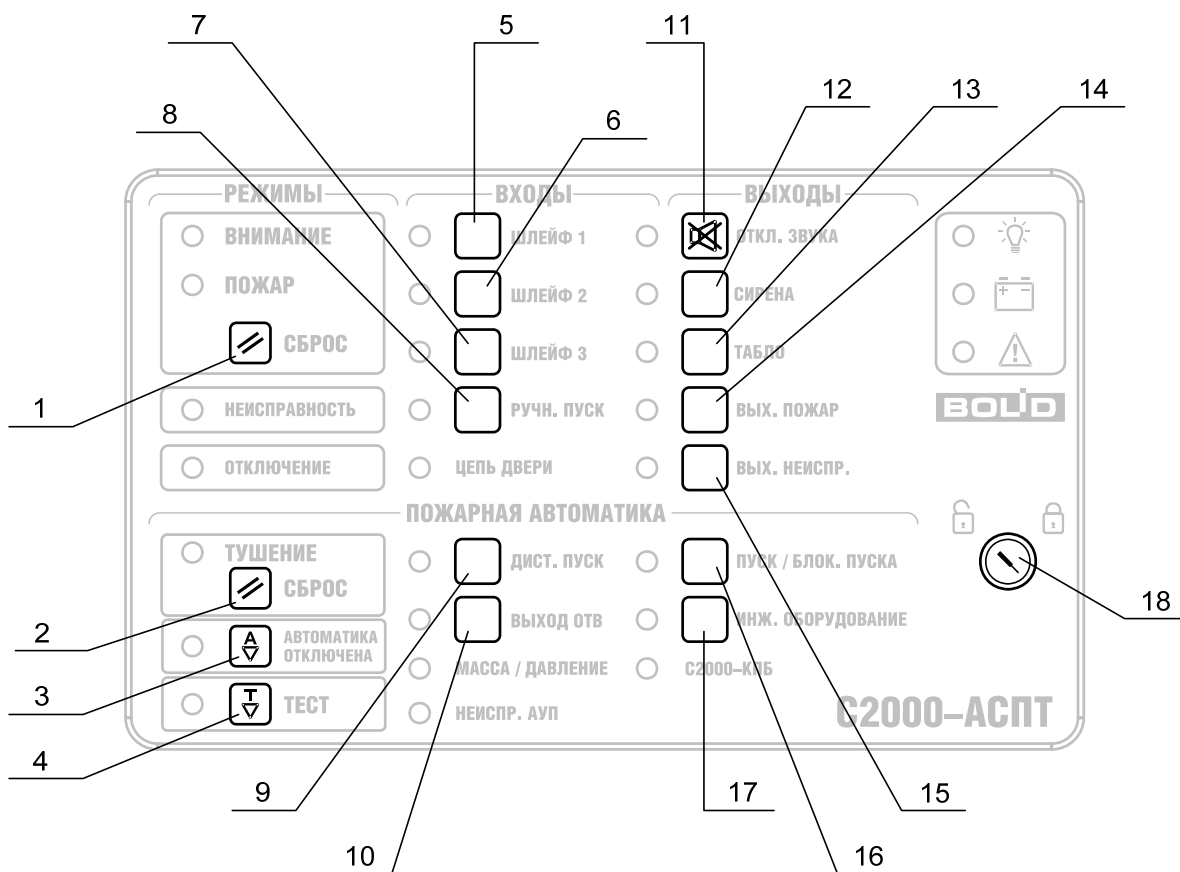
Рисунок 2.2 Расположение кнопок
