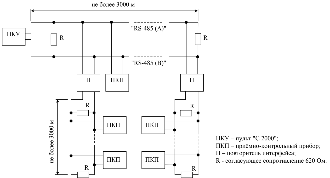
Рисунок 4 Построение конфигурации "звезда" при помощи повторителей интерфейса
