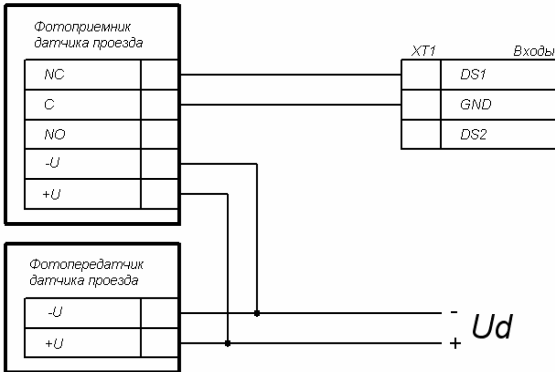
Рисунок 12 Схема подключения датчиков проезда
