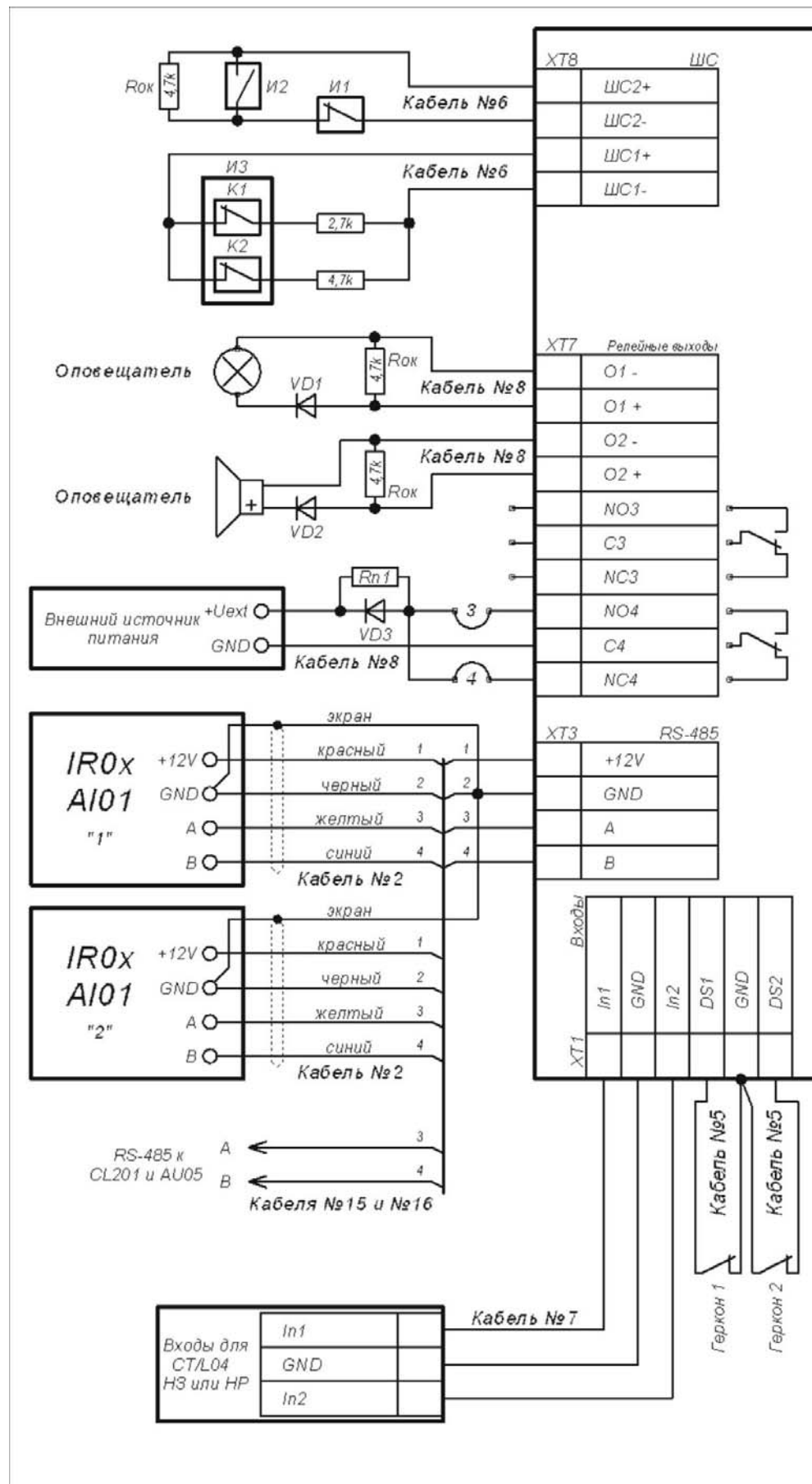
Рисунок 3 Схема подключений
